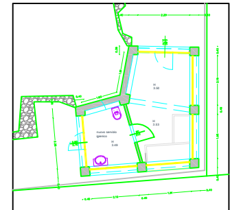
PIANTA
